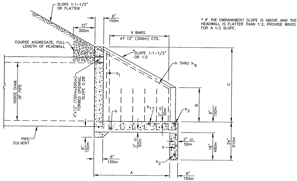
SECTION A-A
