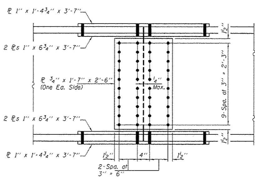
WEB SPLICE
