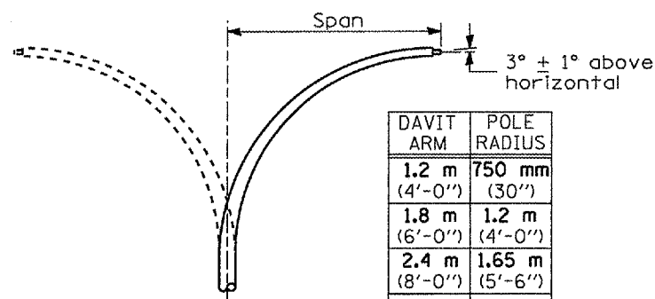
DAVIT ARM
