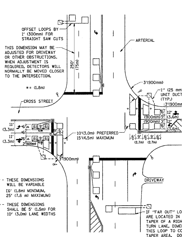
DETAIL 2 N.T.S.
