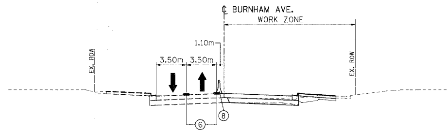
TYPICAL SECTION (STAGE II) STA 59+814.300 TO STA 59+971.200 AND STA 60+030.745 TO STA 60+161.000
