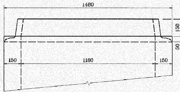
SECTION D-D
