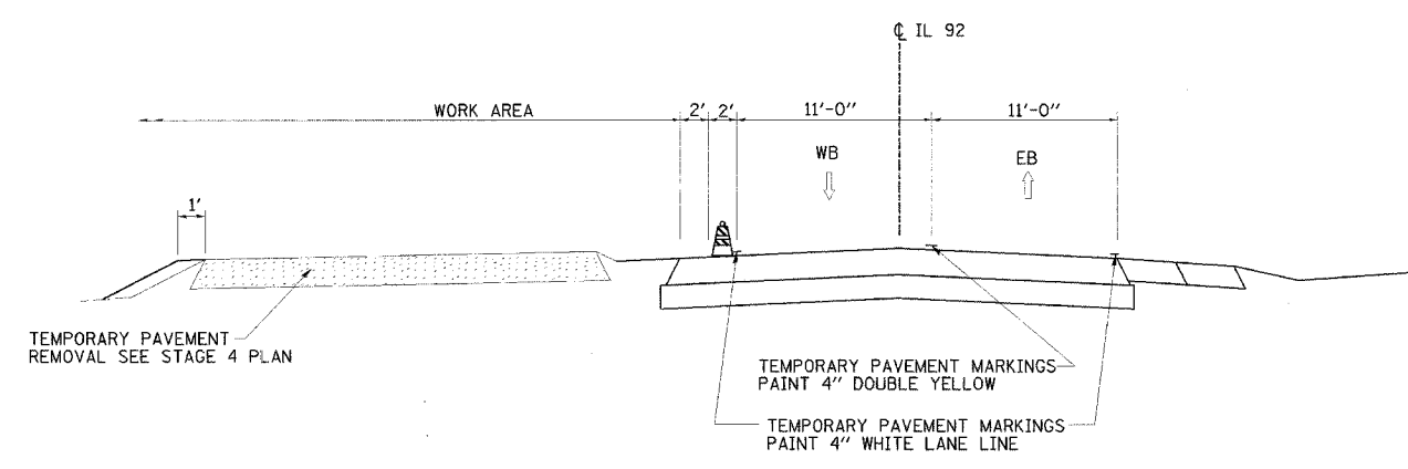
STAGE 4 STA 404+30 TO STA 411+63.5
