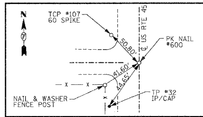
TR1425N STA 10+00.00
