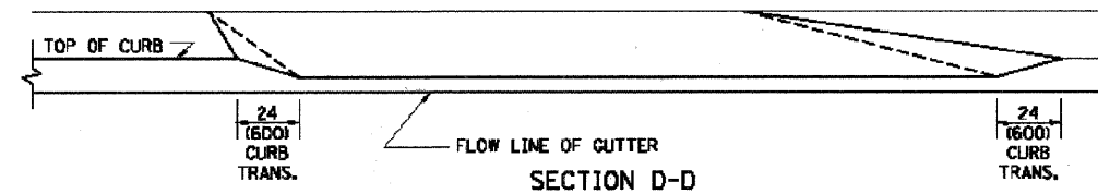
SECTION D-D
