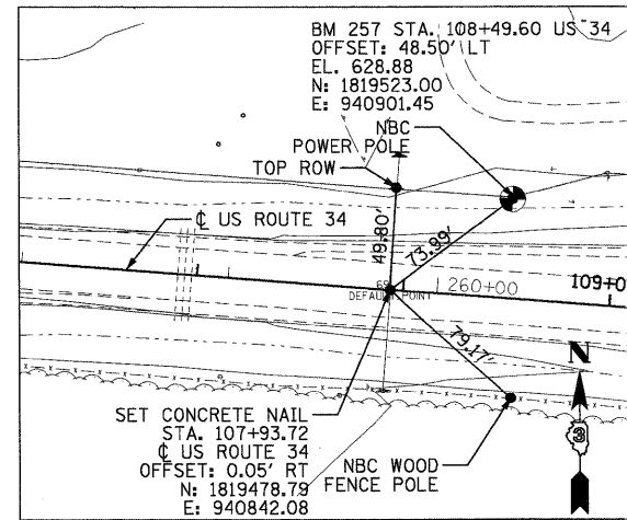
STA. 107+93.72
