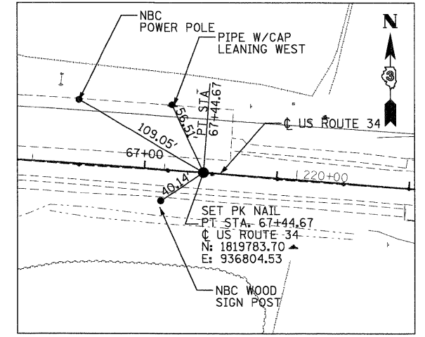
PT STA. 67+44.67
