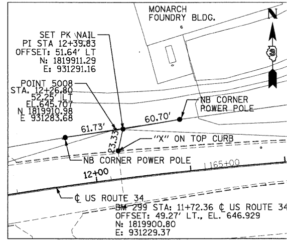
PI STA. 12+39.85
