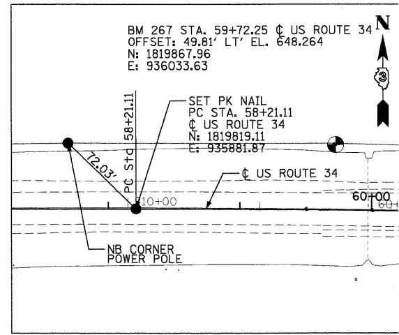
PC STA. 58+21.11
