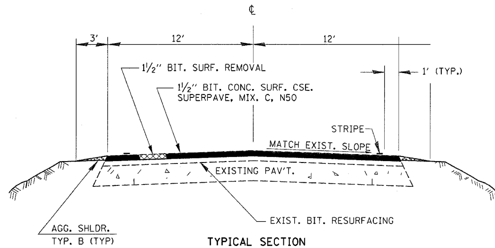
TYPICAL SECTION STA. 3+50 TO STA. 104+10 STA. 111+40 TO STA. 458+62
