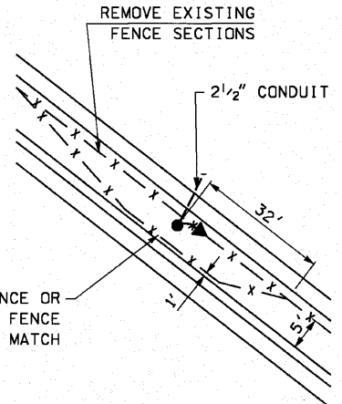
FENCE DETAIL N.T.S.
