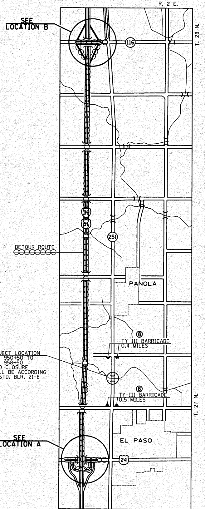
DETOUR PLAN
