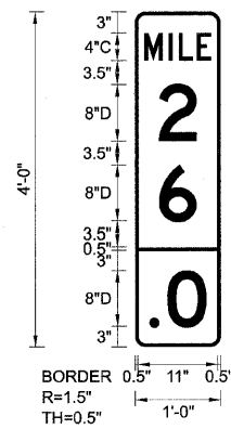
EB-MM-53 STA. 1012+20
