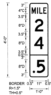
EB-MM-50 STA. 933+00
