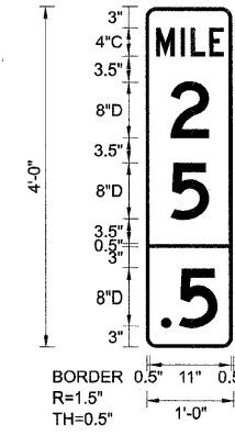
EB-MM-52 STA. 985+80
