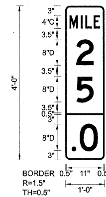
EB-MM-51 STA. 959+40
