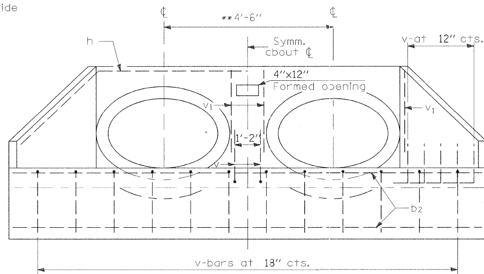
END ELEVATION
