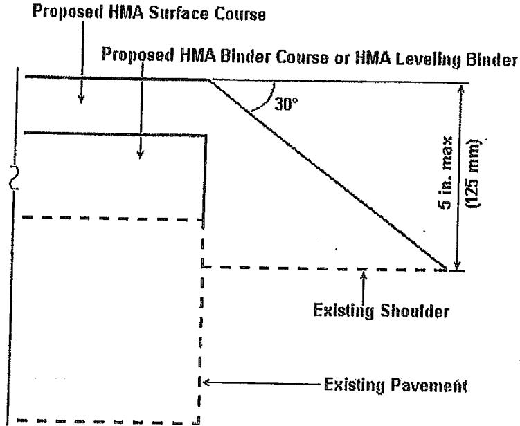
Safety Edge at Edge of Pavement
