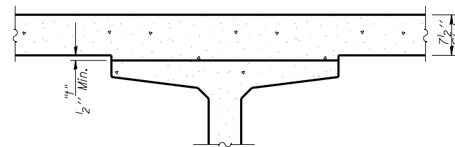
FILLET HEIGHTS
