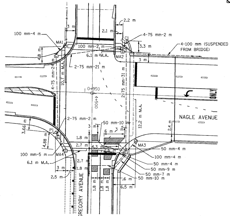
FOUNDATION & CONDUIT PLAN SCALE: 1=250
