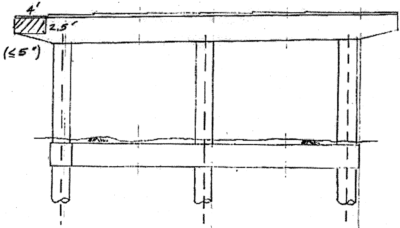
PIER # 10 - N. END / W. FACE - (W11)
