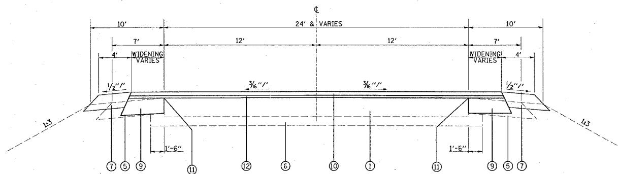
STA. 238+38.00 TO STA. 239+50.00
