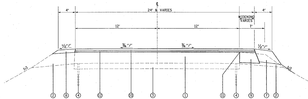
STA. 239+89.00 TO STA. 241+20.00
