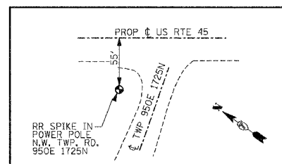
BENCHMARK #19 STA 1006+18 ELEVATION 512.53
