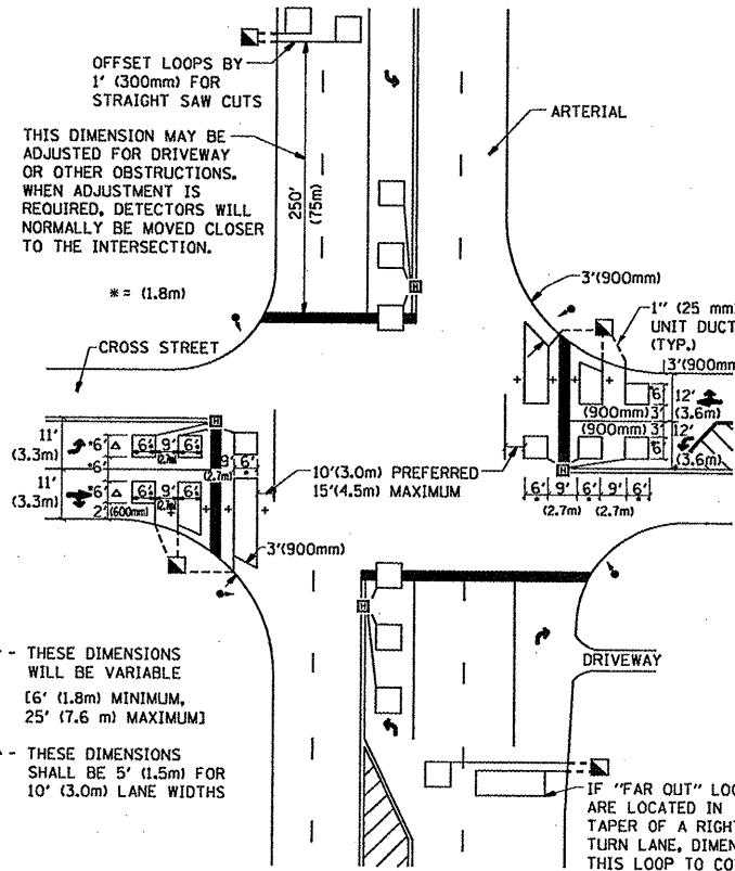
DETAIL 2 N.T.S.
