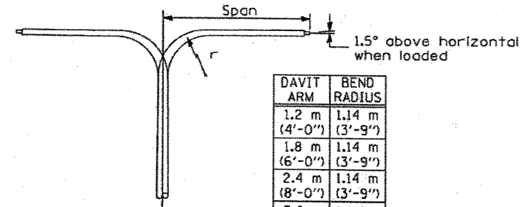
DAVIT ARM
