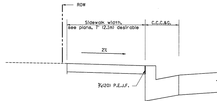
SECTION D-D
