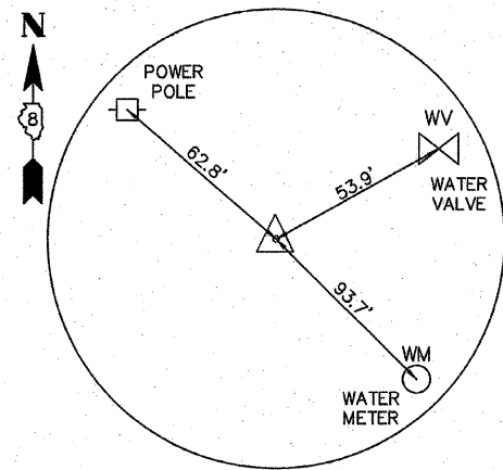
O'FALLON-TROY ROAD POT STA 239+02.50
