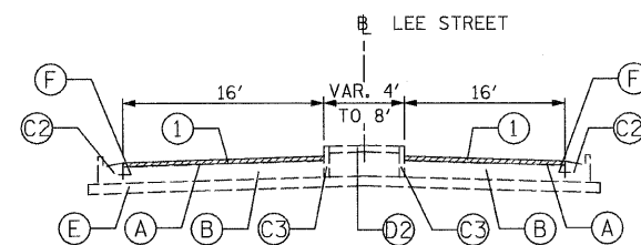
EXISTING TYPICAL SECTION STA. 300+32 TO STA. 303+10
