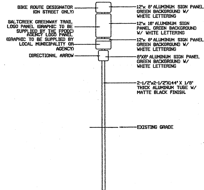
A6 TRAIL MARKER D1.0 ELEVATION - N.T.S.
