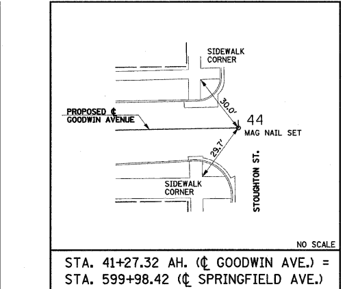
STA. 41+27.32 AH. (CL GOODWIN AVE.) = STA. 599+98.42 (CL SPRINGFIELD AVE.)
