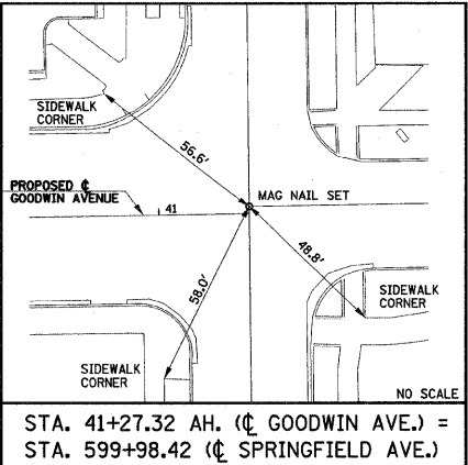
STA. 41+27.32 AH. (CL GOODWIN AVE.) = STA. 599+98.42 (CL SPRINGFIELD AVE.)
