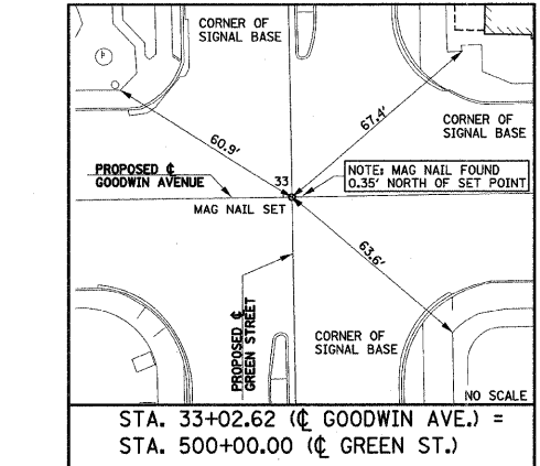
STA. 33+02.62 (CL GOODWIN AVE.) = STA. 500+00.00 (CL GREEN ST.)
