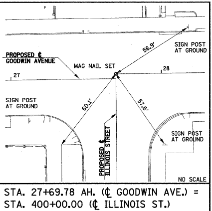
STA. 27+69.78 AH. (CL GOODWIN AVE.) = STA. 400+00.00 (CL ILLINOIS ST.)
