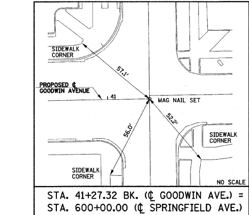
STA. 41+27.32 BK. (CL GOODWIN AVE.) = STA. 600+00.00 (CL SPRINGFIELD AVE.)
