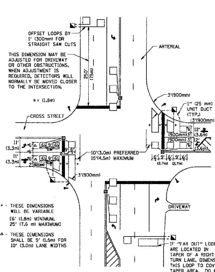
DETAIL 2 N.T.S.
