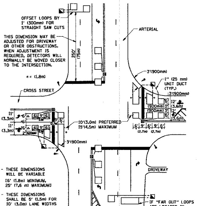
DETAIL 2 N.T.S.
