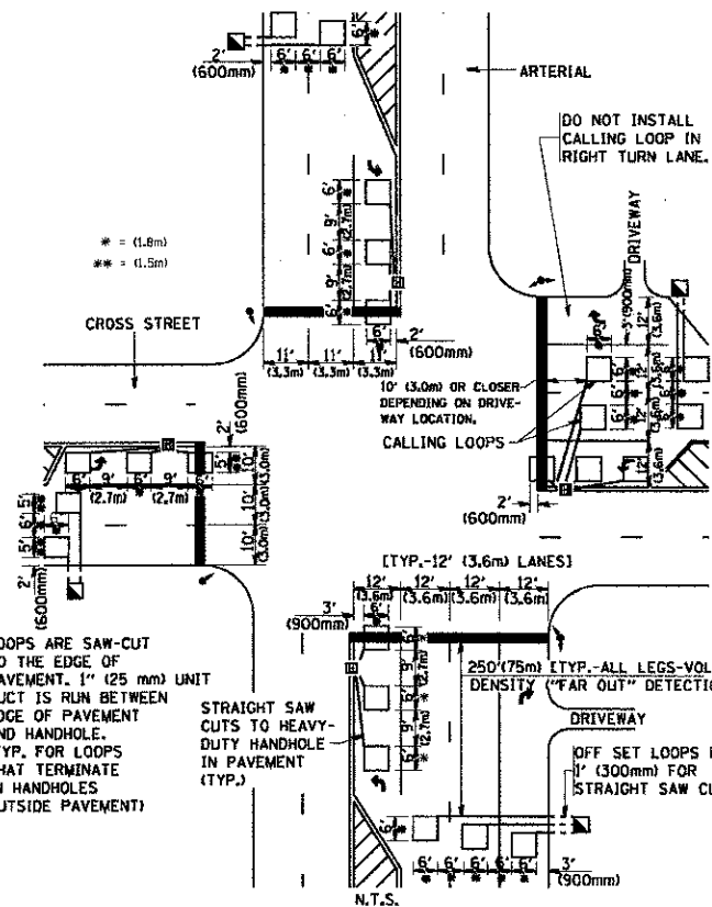
DETAIL 1 N.T.S.
