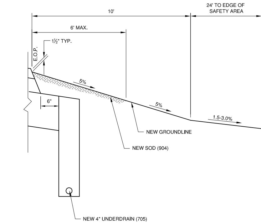
NEW SHOULDER DETAIL "A" N.T.S.
