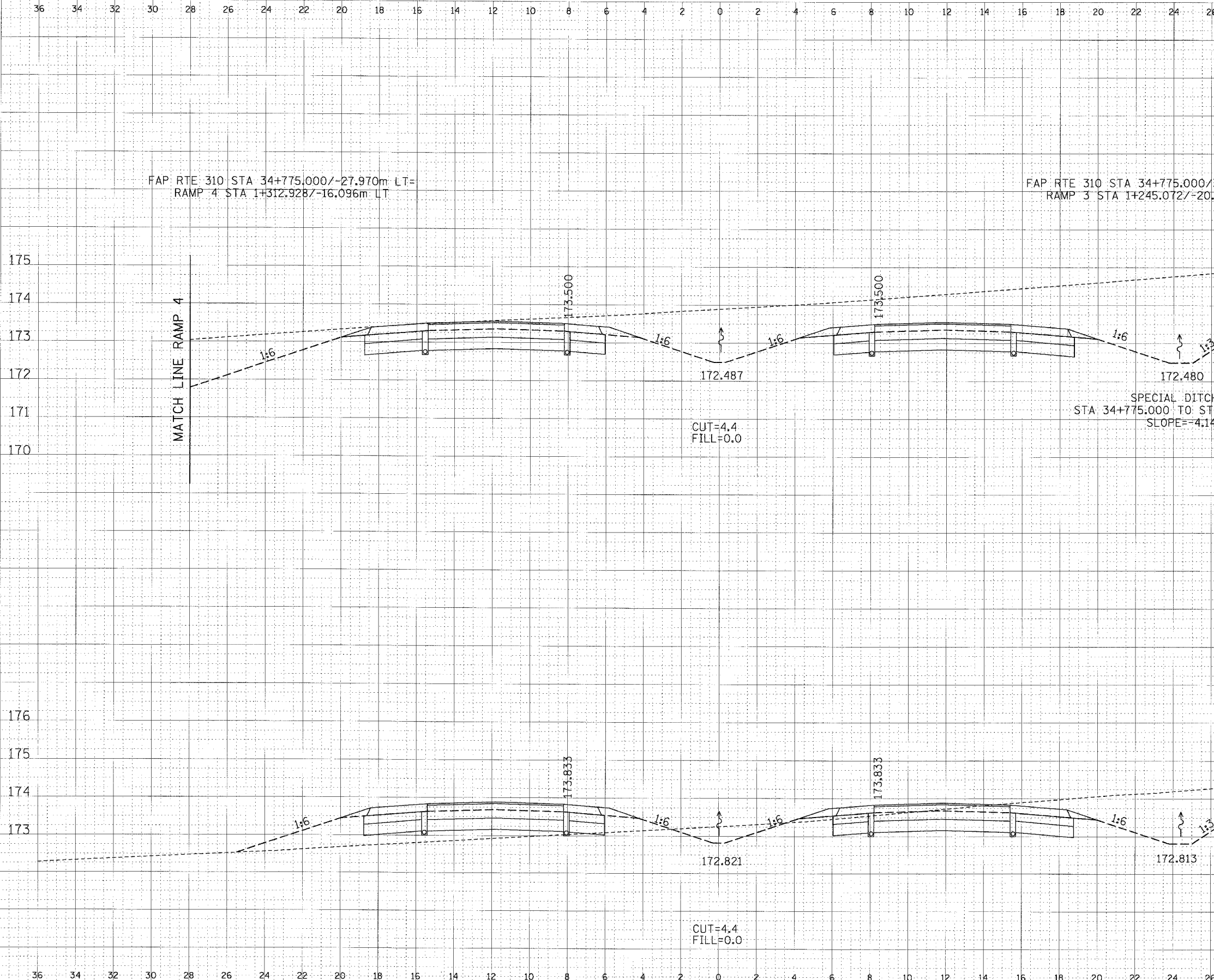
CROSS SECTION, FAP ROUTE 310, STA 34+750.000 TO STA 34+775.000
