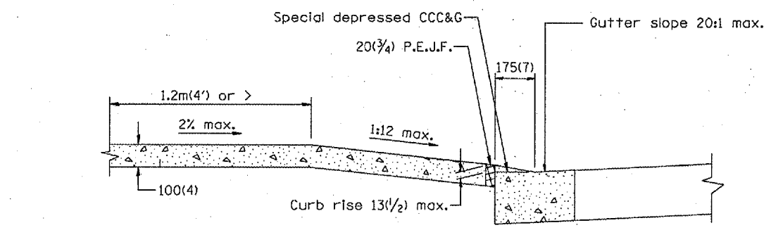
SEC. A-A
