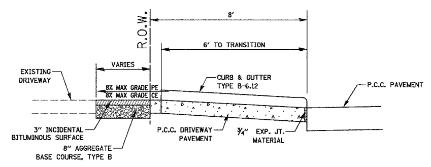
SECTION A-A 2 N.T.S.
