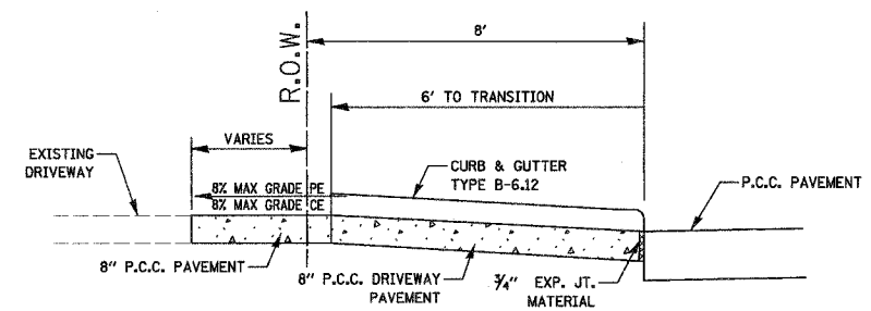
SECTION A-A 1 N.T.S.
