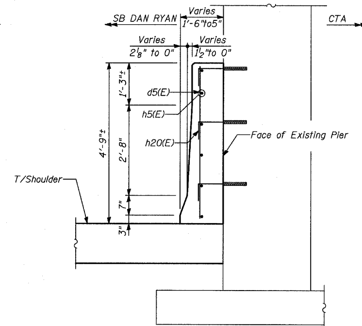
SECTION D-D
