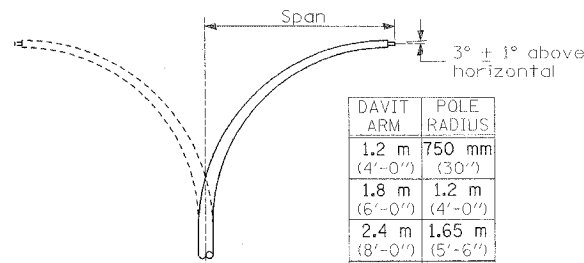
DAVIT ARM
