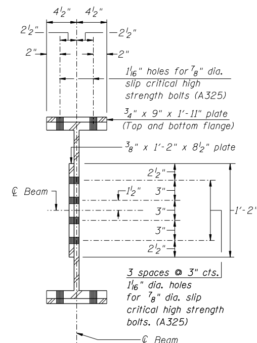
SECTION A-A (Option 2)
