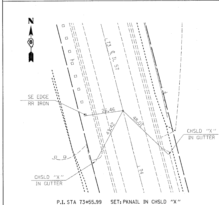
P.I. STA 73+55.99 SET: PKNAIL IN CHSLD "X"
