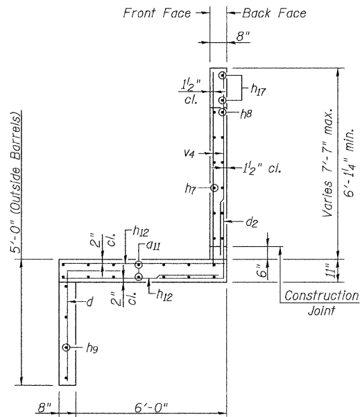
SECTION D-D
