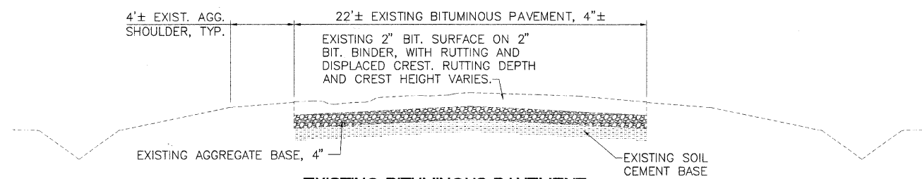
EXISTING BITUMINOUS PAVEMENT STA. 349+34.19 BACK = 353+35.81 AHEAD TO STA. 359+00 STA. 373+50 TO STA. 375+81.81 STA. 379+15.35 TO STA. 381+50 STA. 414+50 TO STA. 418+23
