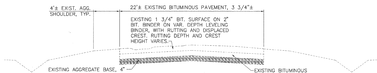
EXISTING BITUMINOUS PAVEMENT STA. 359+00 TO STA. 373+50 STA. 381+50 TO STA. 414+50
