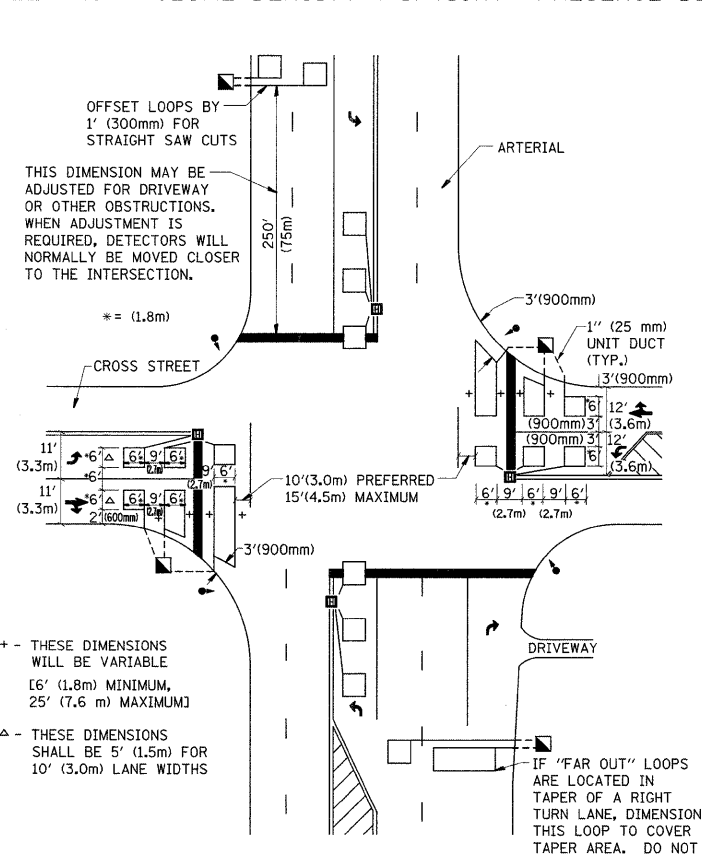
DETAIL 2 N.T.S.
