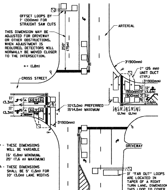
DETAIL 2 N.T.S.
