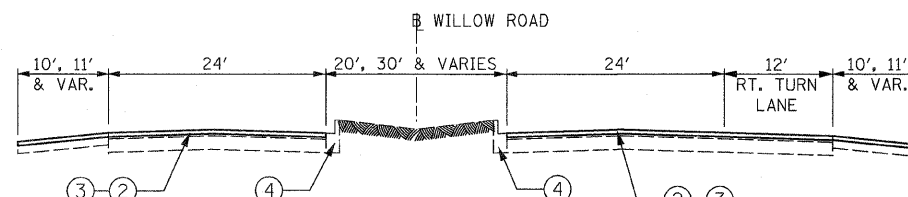
PROPOSED TYPICAL SECTION STA. 57+40 TO STA. 60+75 STA. 70+30 TO STA. 73+15
