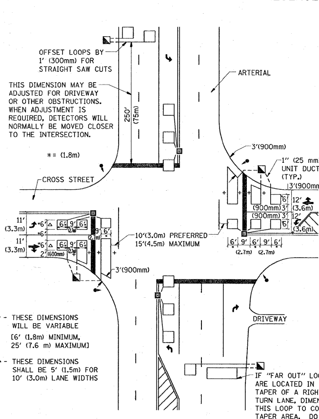
DETAIL 2 N.T.S.
