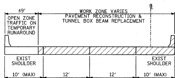
YY-YY
