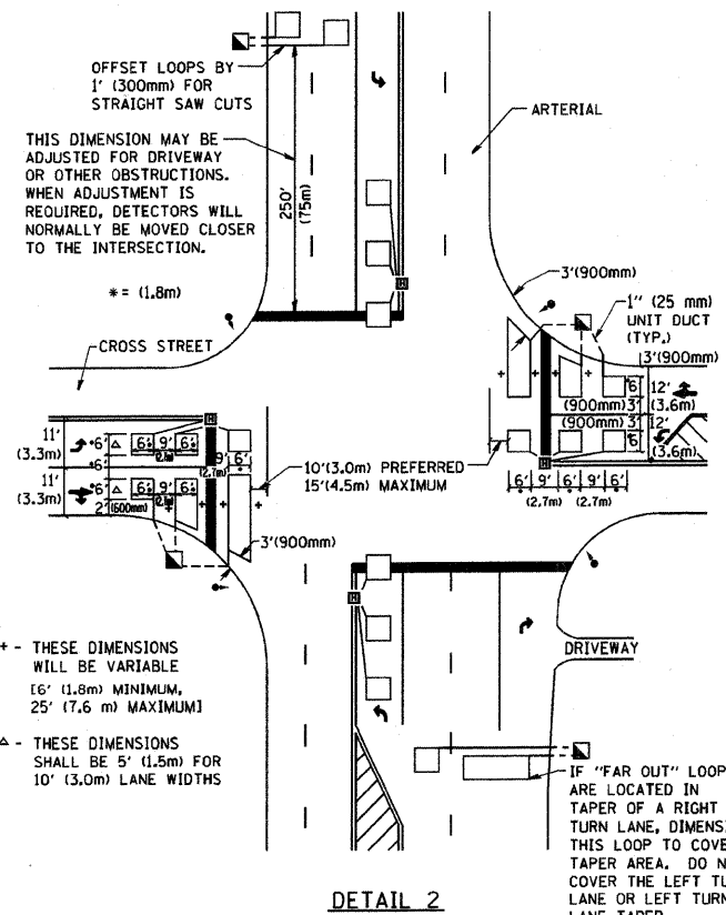
DETAIL 2 N.T.S.
