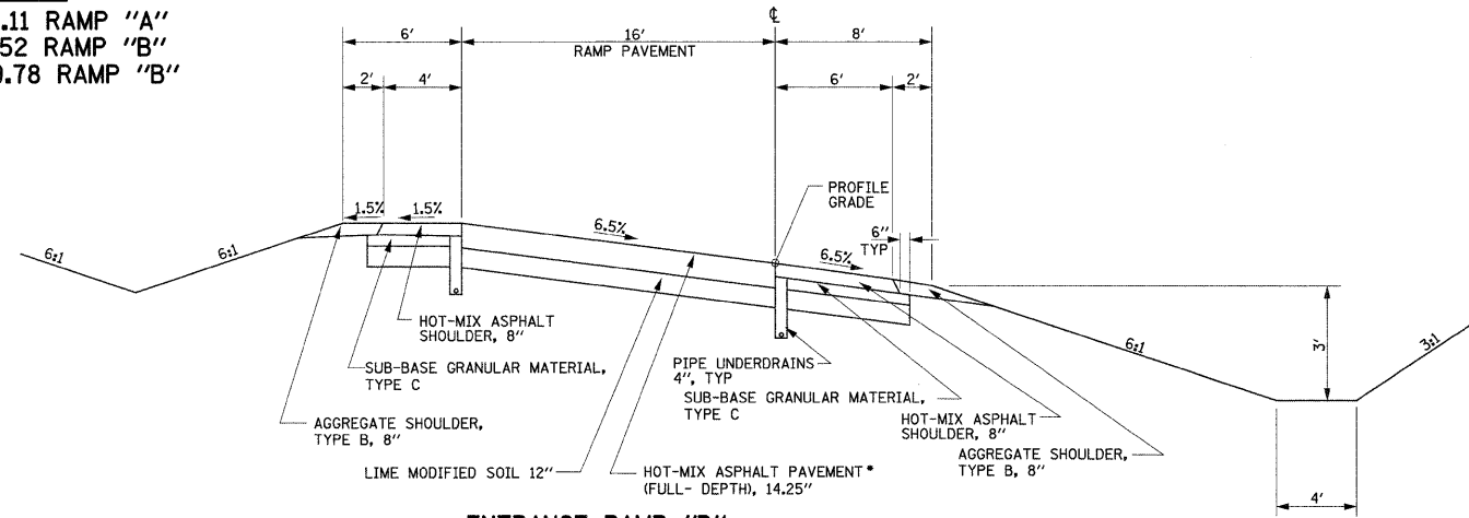
ENTRANCE RAMP "B" STA 31+08.68 TO STA 34+25.49
