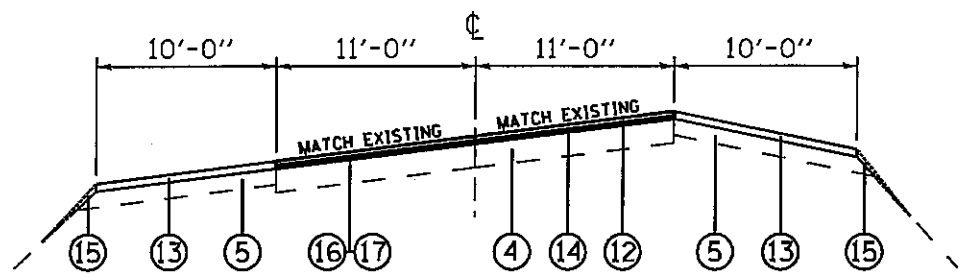
TYPICAL SECTION STA. 84+29.15 TO STA. 89+22.83 STA. 111+06.06 TO STA. 118+33.17
