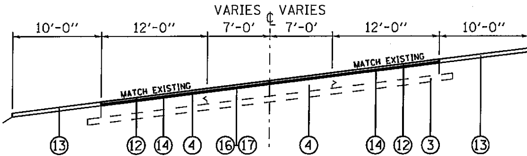
TYPICAL SECTION STA 22+70.32 TO STA. 30+75
