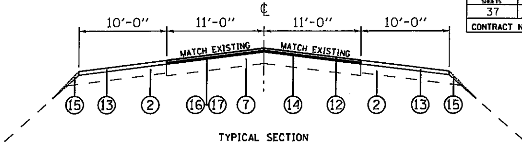
TYPICAL SECTION STA. 83+40 TO STA. 84+29.15 STA. 118+33.17 TO STA. 121+29.72 STA. 189+88.88 TO STA. 191+85.00 STA. 192+77.50 TO STA. 199+77.66
