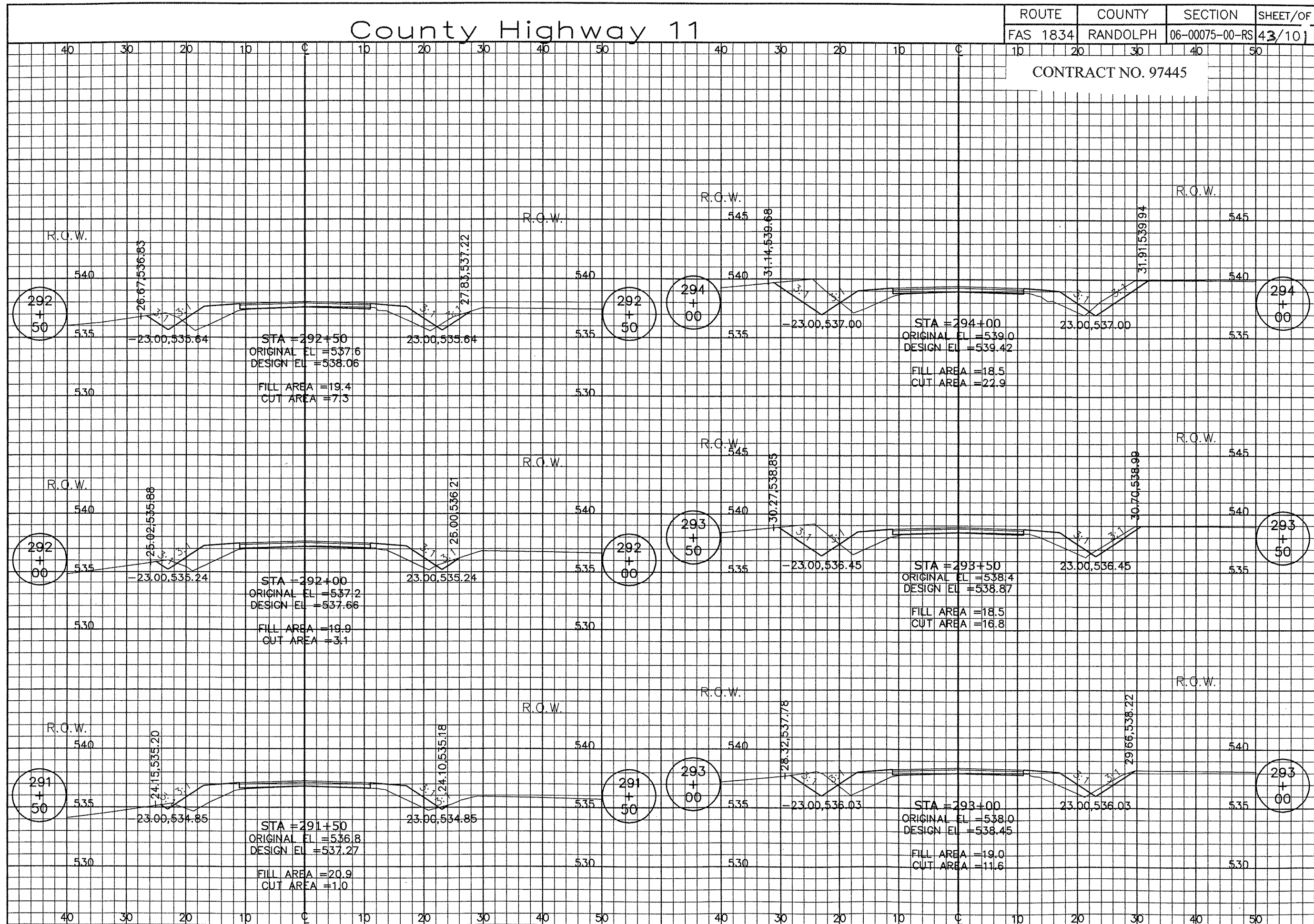
CROSS SECTIONS STA. 291+50 TO STA. 294+00
