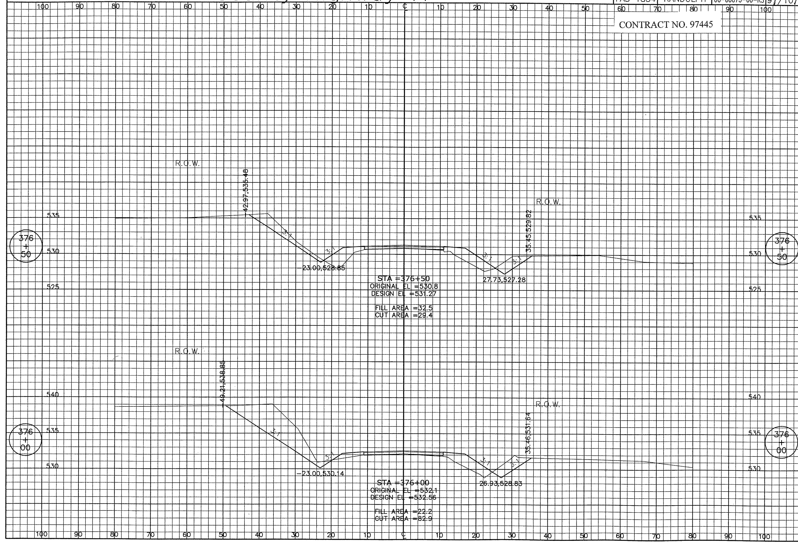
CROSS SECTIONS STA. 376+00 TO STA. 376+50
